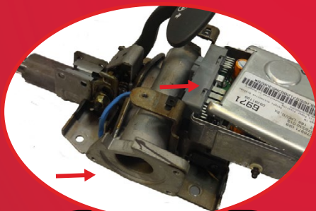
Poškozený, demontovaný nebo chybějící motor nebo ECU
