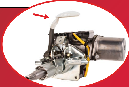
Prasklá rukojeť pro nastavení výšky
