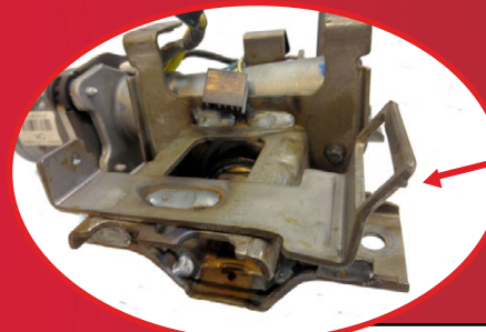
Poškozený nebo ohnutý montážní rám
